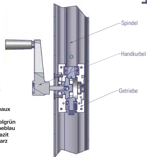
Ansicht B
