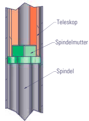
Ansicht A
