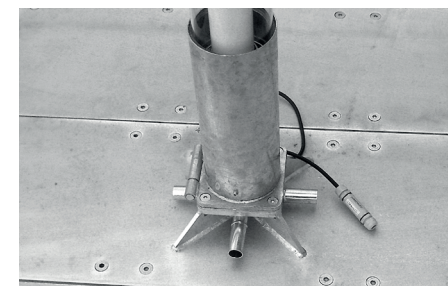
Verankerung 3 x 3 m Anchoring 3 x 3 m
