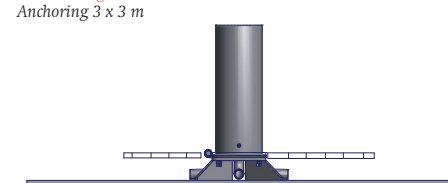
Verankerung 3 x 3 m Anchoring 3 x 3 m
